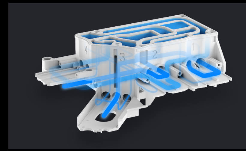
立体集成水路
