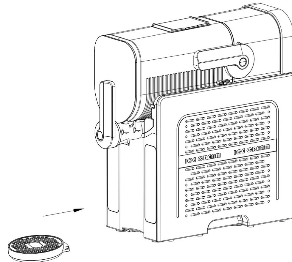
5.拆下杯盘
