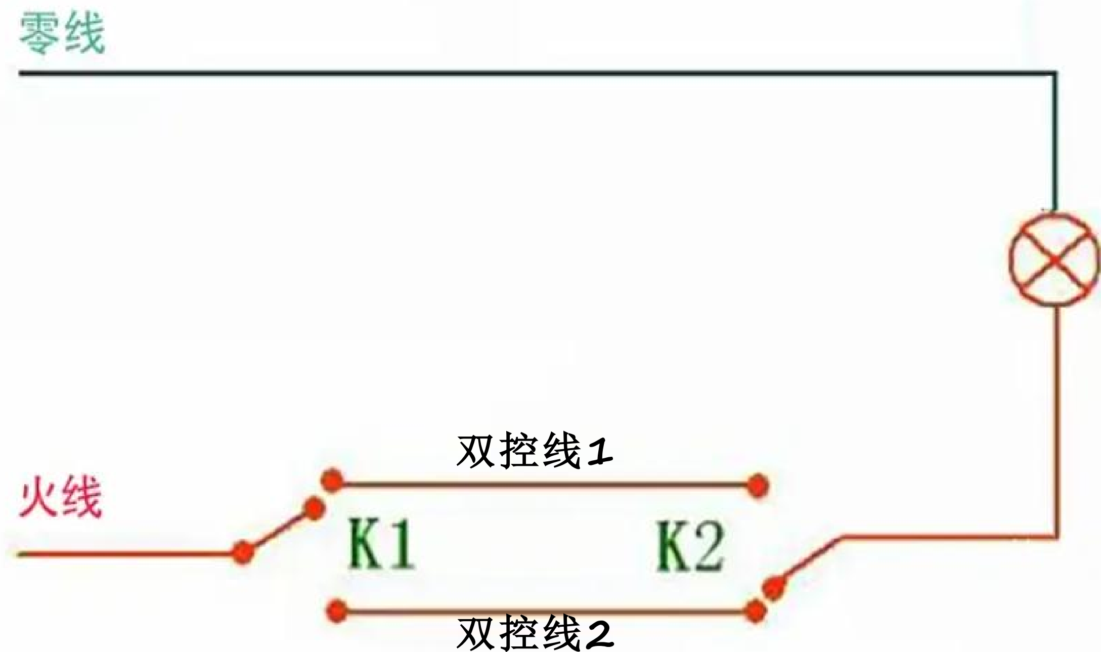
传统双控开关常规接线
