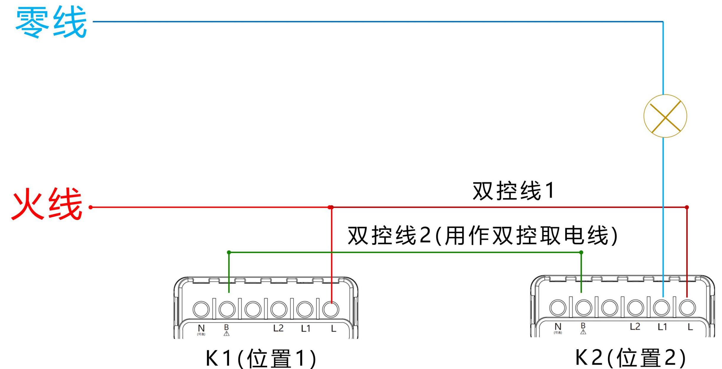
云米Super开关，单火双控利用原双控线
