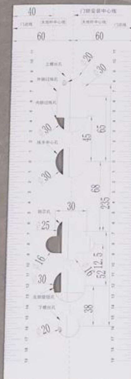
安装 开孔图
